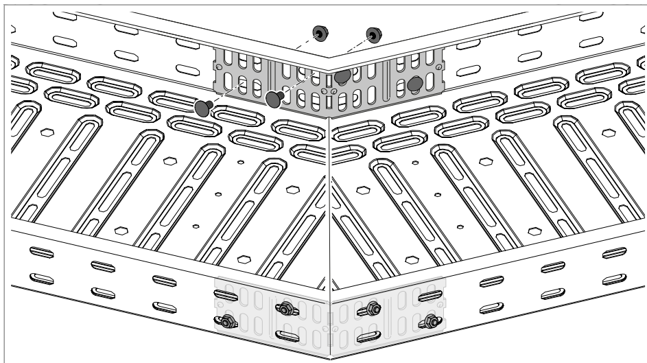
35 pav. Kampinio sujungimo elemento RWVL prisukimas
