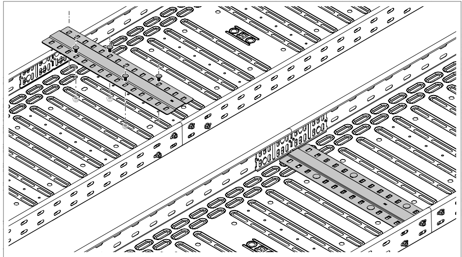
16 pav. Sandūros juostelės montavimas
