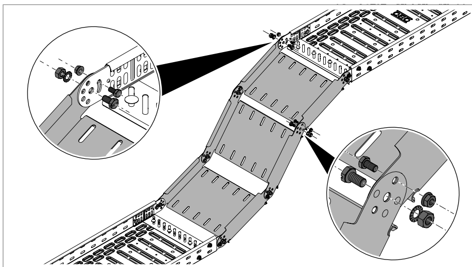
72 pav. Lankstinių dugno elementų montavimas
