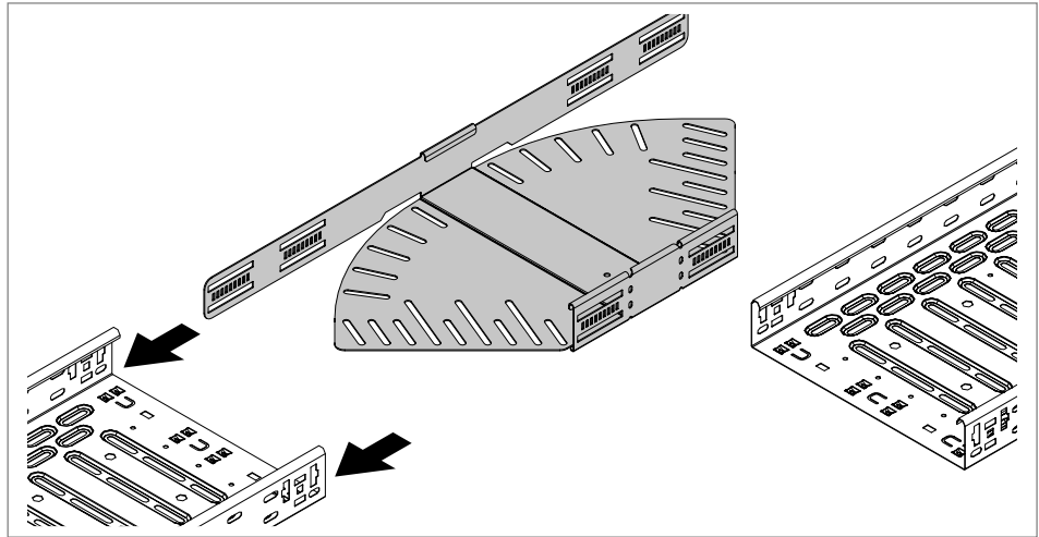
60 pav. Reguliuojamo kampo alkūnės įstūmimas
