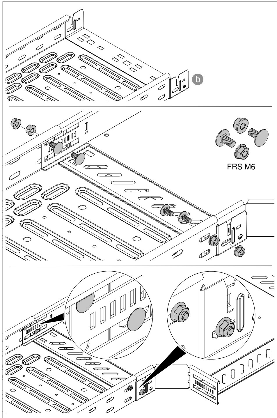
49 pav. Fasoninės dalies pritvirtinimas varžtais (Kabelių lovio galas (b))
