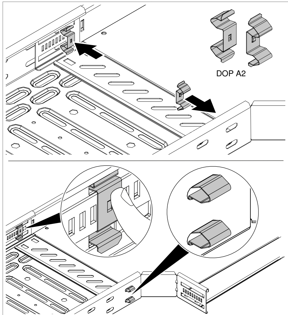
51 pav. Fasoninės dalies pritvirtinimas dvigubu gnybtu
