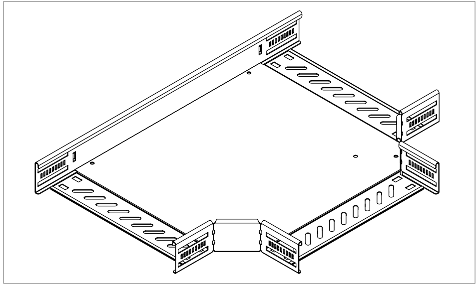
6 pav. T formos detalė
