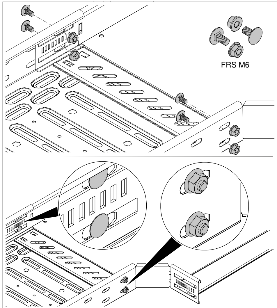
53 pav. Fasoninės dalies pritvirtinimas dvigubu gnybtu
