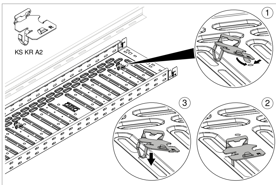
79 pav. Pertvaros fiksatoriaus įstatymas
