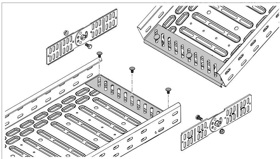
39 pav. Pagrindo galinių plokščių priveržimas
