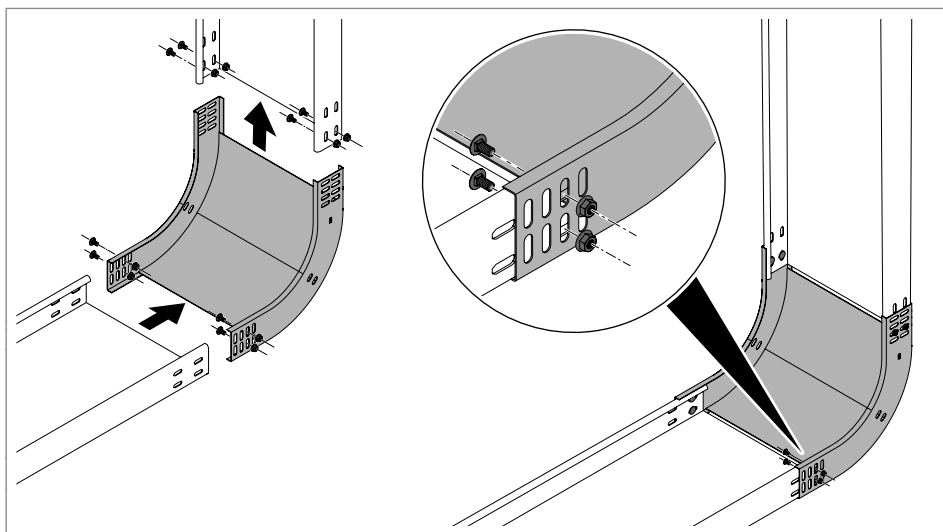
68 pav. Besileidžiančios vertikaliosios alkūnės montavimas
