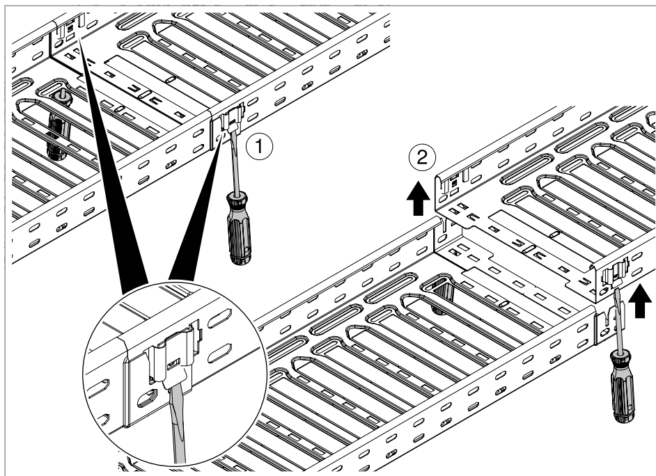
92 pav. Fiksuojamosios jungties „Magic“ pakartotinis atlaisvinimas
