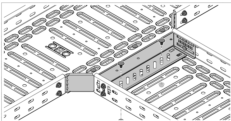
57 pav. Atšakinio kabelių lovio prisukimas prie primontuojamosios atšakos
