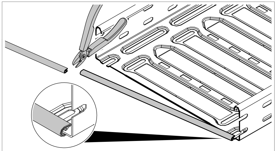
17 pav. Briaunų apsauginės juostos uždėjimas
