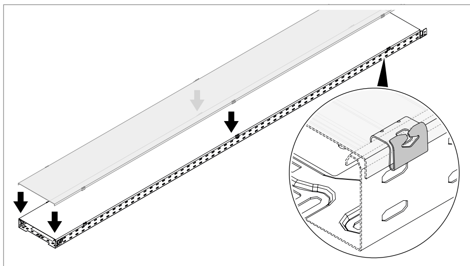
85 pav. Dangčio užfiksavimas
