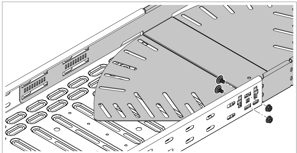
61 pav. Reguliuojamo kampo alkūnės užfiksavimas
