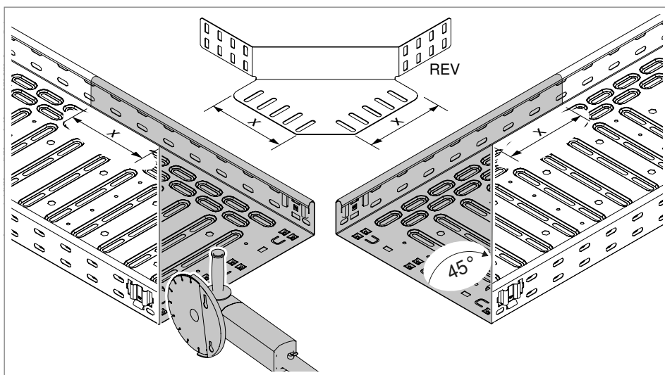
36 pav. Kabelių lovių pjaustymas kampo sujungimo elementui REV
