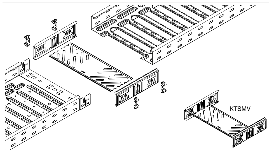
21 pav. Išilginis sujungimo elementas KTSM
