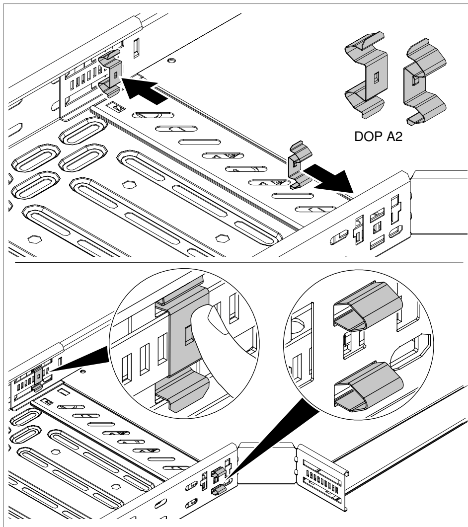
46 pav. Fasoninės dalies pritvirtinimas dvigubu gnybtu
