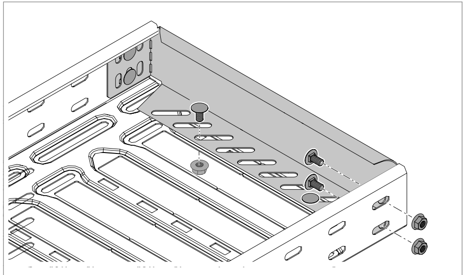
77 pav. Galinio elemento montavimas
