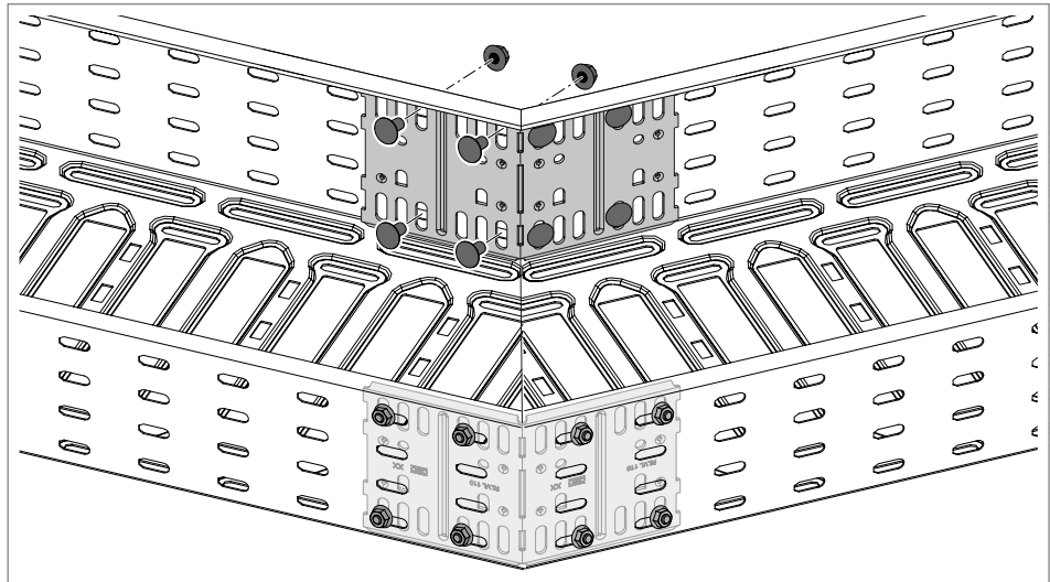
32 pav. Išilginio ir kampinio sujungimo elemento RLVL prisukimas
