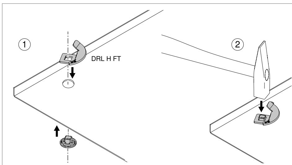
88 pav. Sukamosios sklendės tvirtinimas kniedėmis
