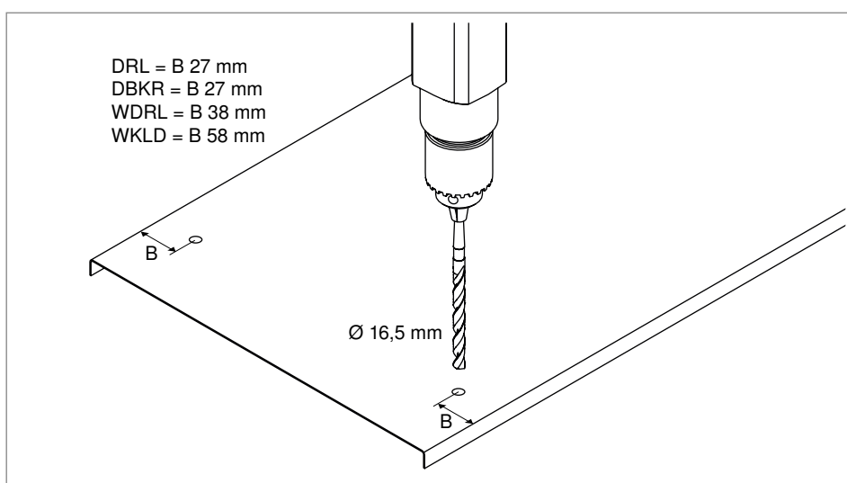
86 pav. Skylių gręžimas dangtyje
