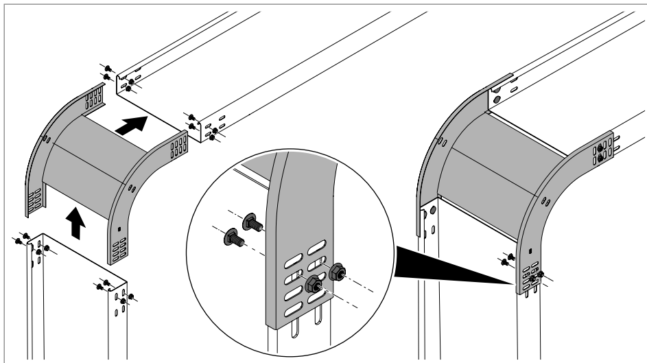
67 pav. Besileidžiančios vertikaliosios alkūnės montavimas
