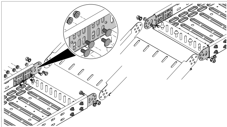
71 pav. Lankstinio sujungimo elemento montavimas prie kabelių lovių
