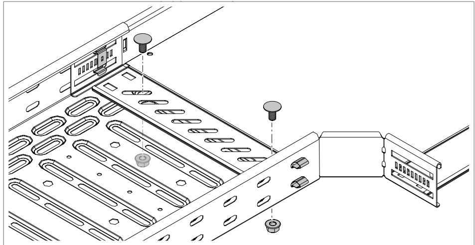
52 pav. Sandūros juostelės prisukimas
