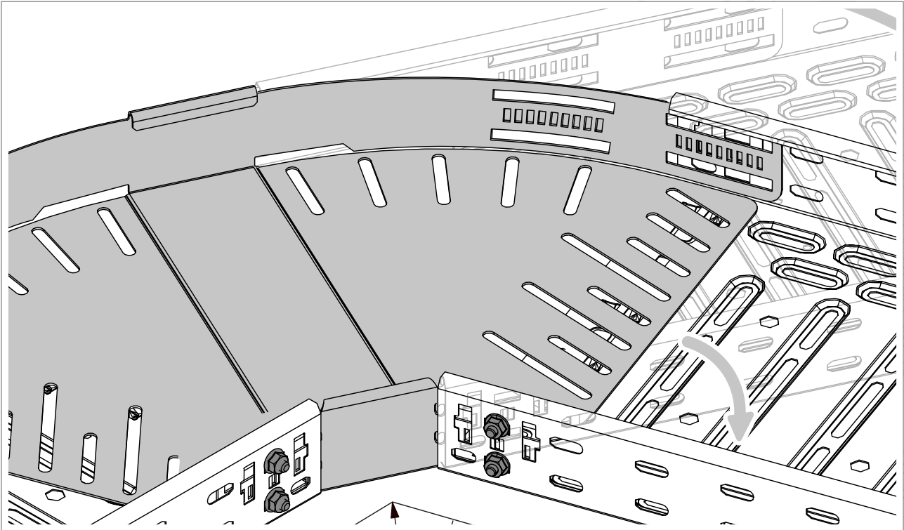
Abb. 65: Lovio užlenkimas ant vidinio sujungimo elemento
