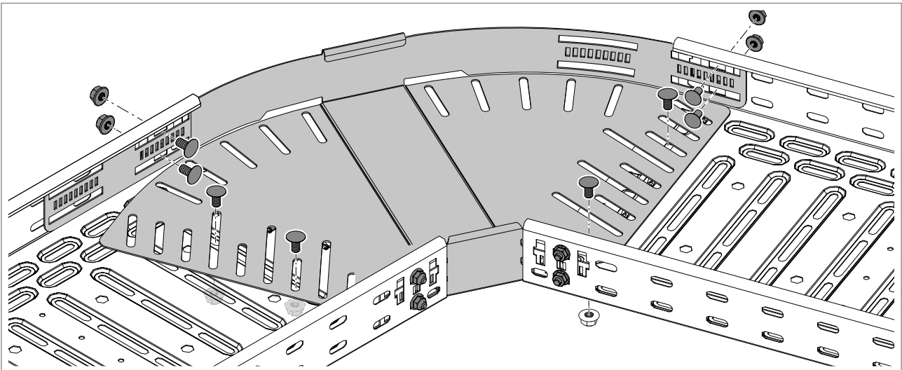
Abb. 66: Lovio sujungimo elemento ir sandūrų prisukimas
