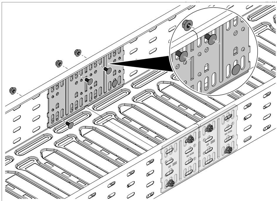
29 pav. Išilginio sujungimo elemento RLVL prisukimas
