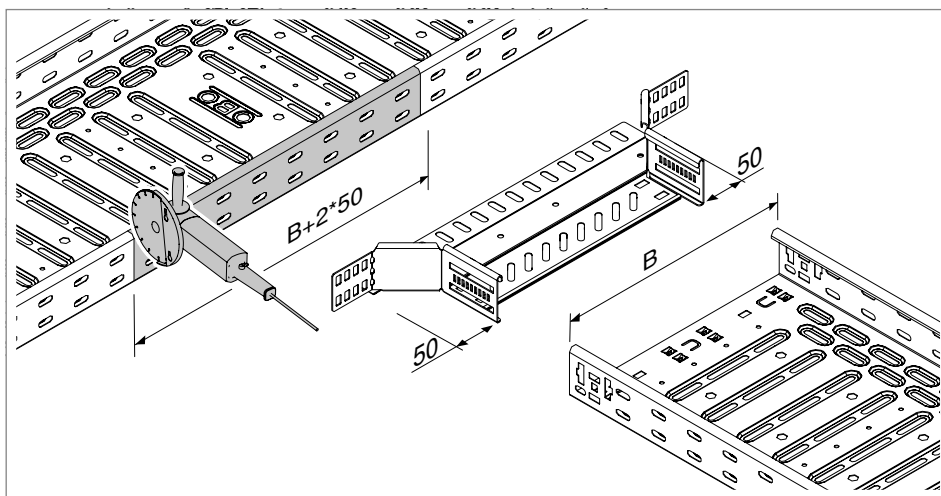
55 pav. Kabelių lovio sienelės išpjovimas
