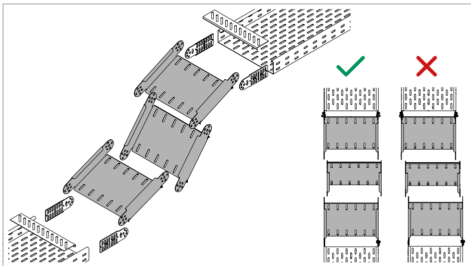
69 pav. Lankstinis alkūninis elementas su puse lankstinio sujungimo elemento ir pagrindo galine plokšte
