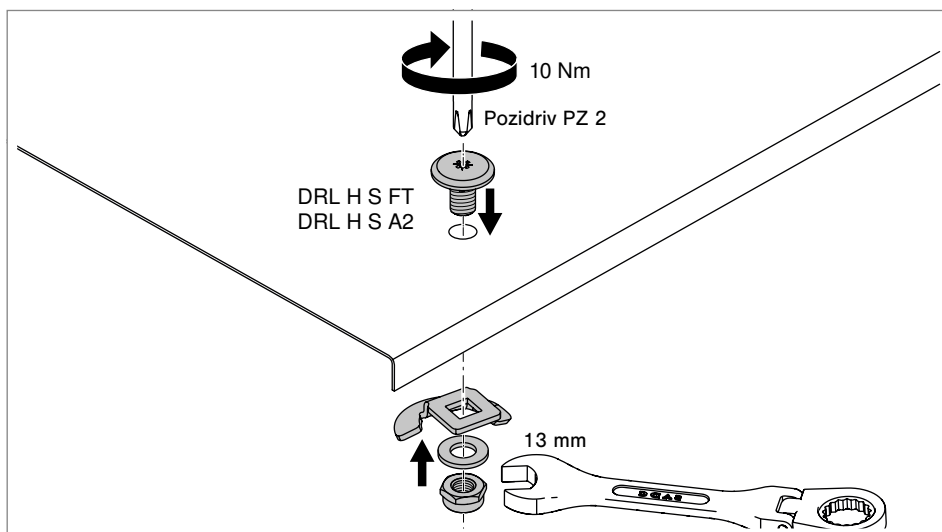
87 pav. Sukamosios sklendės prisukimas
