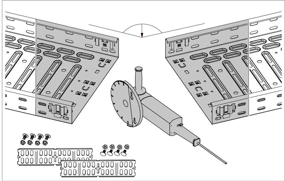
33 pav. Kabelių lovio nupjovimas kampu
