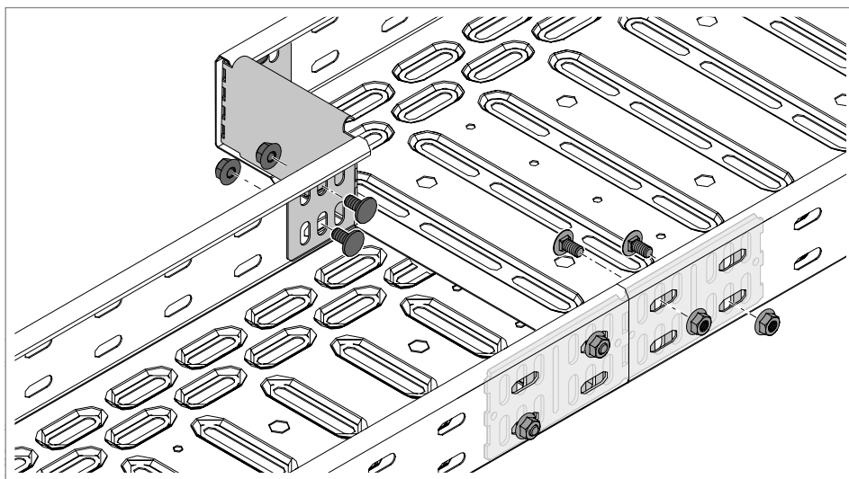
74 pav. Išilginio ir kampinio sujungimo elemento bei pereinamojo kampinio elemento montavimas
