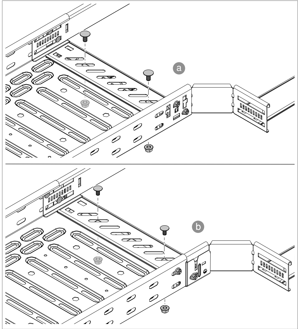
50 pav. Sandūros juostelės prisukimas (Kabelių lovio galas a ir b )
