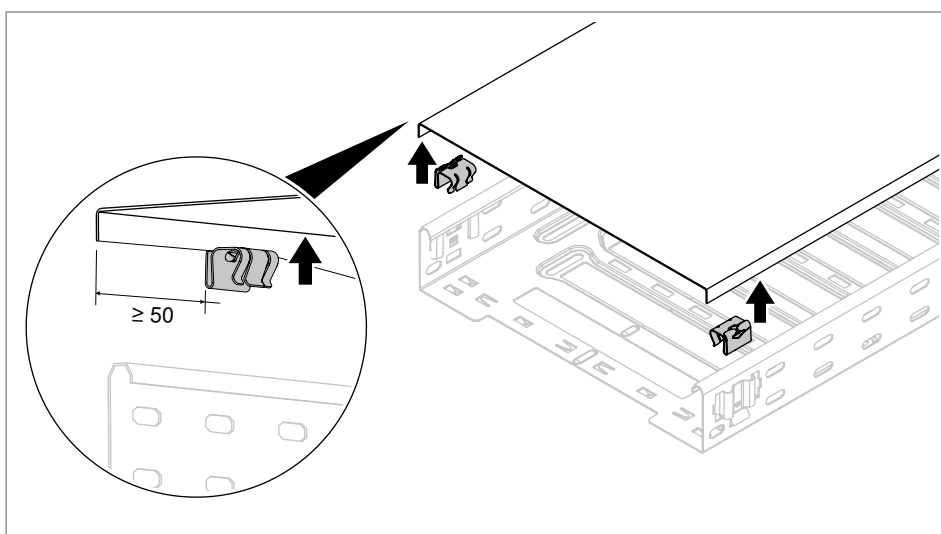
83 pav. Dangčio spaustuvių užspaudimas
