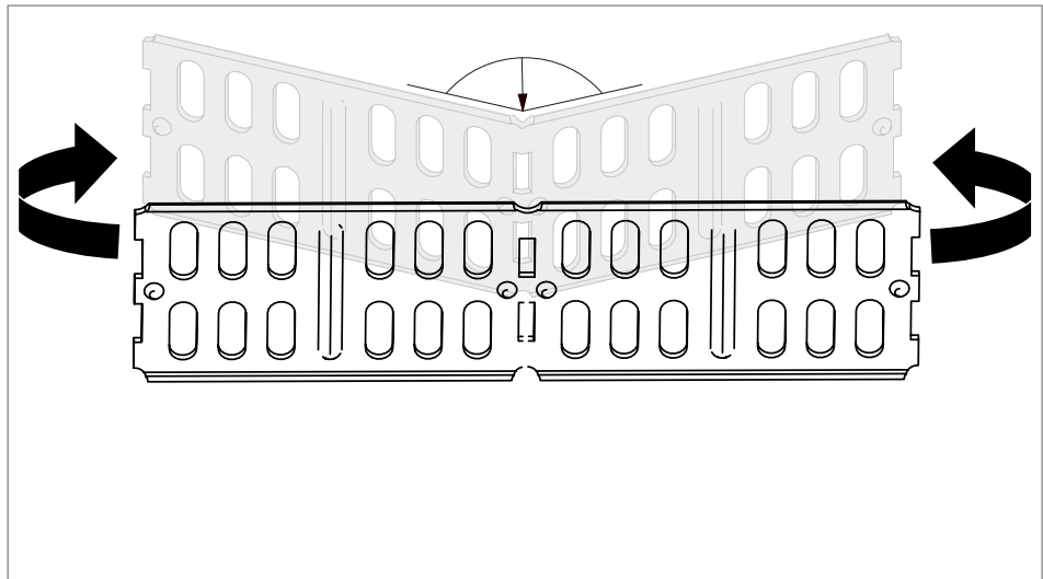
34 pav. Kampinio sujungimo elemento RWVL užlenkimas
