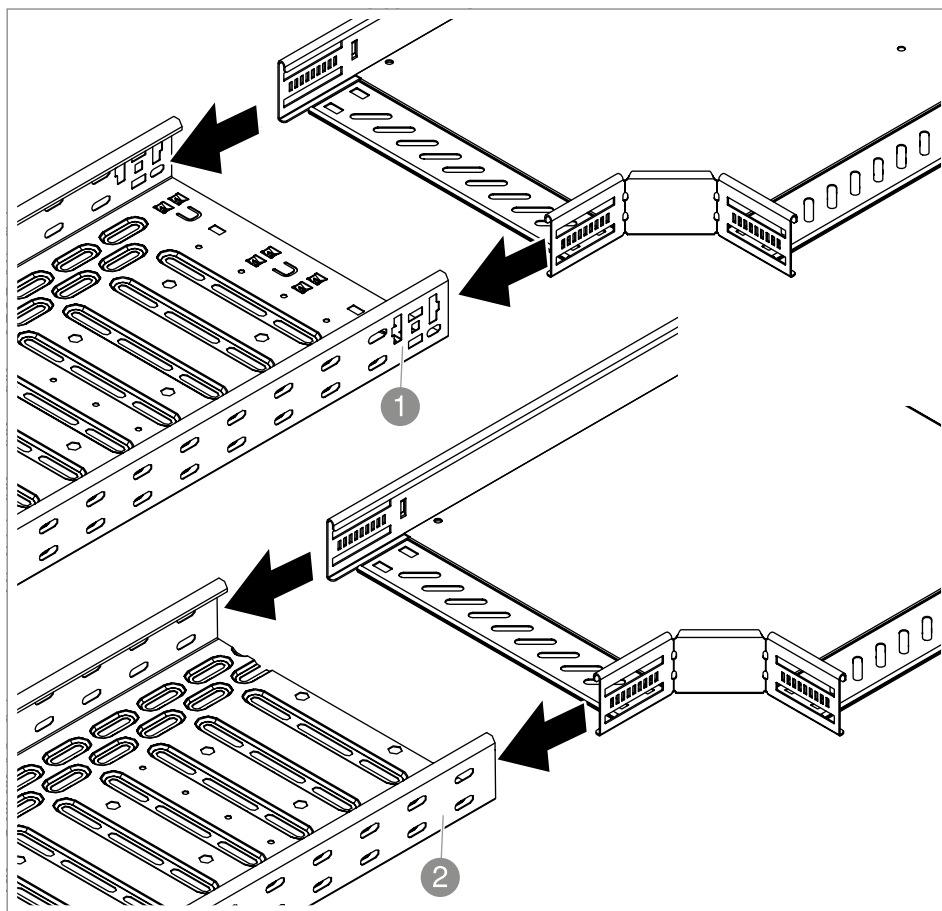
45 pav. Fasoninės dalies įstūmimas
