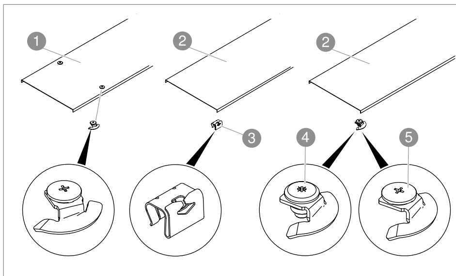
10 pav. Dangtis su tvirtinimo medžiaga kabelių loviams
