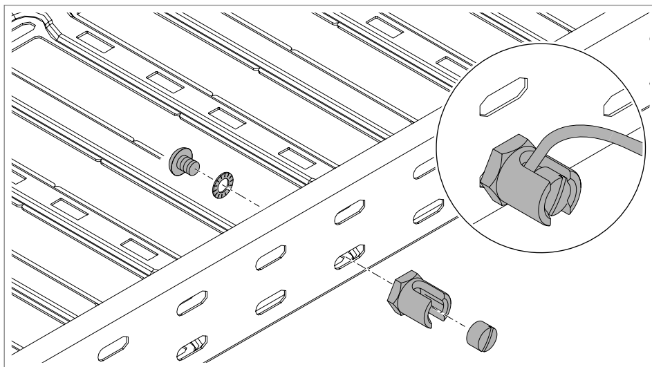
82 pav. Įžeminimo gnybto montavimas
