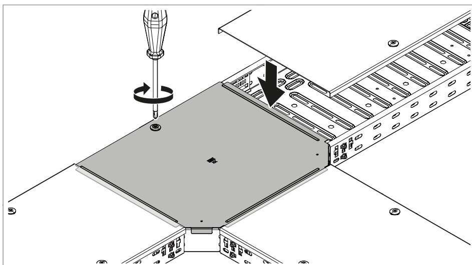
91 pav. Fasoninių dalių dangčio užfiksavimas atkarpos dangčiu
