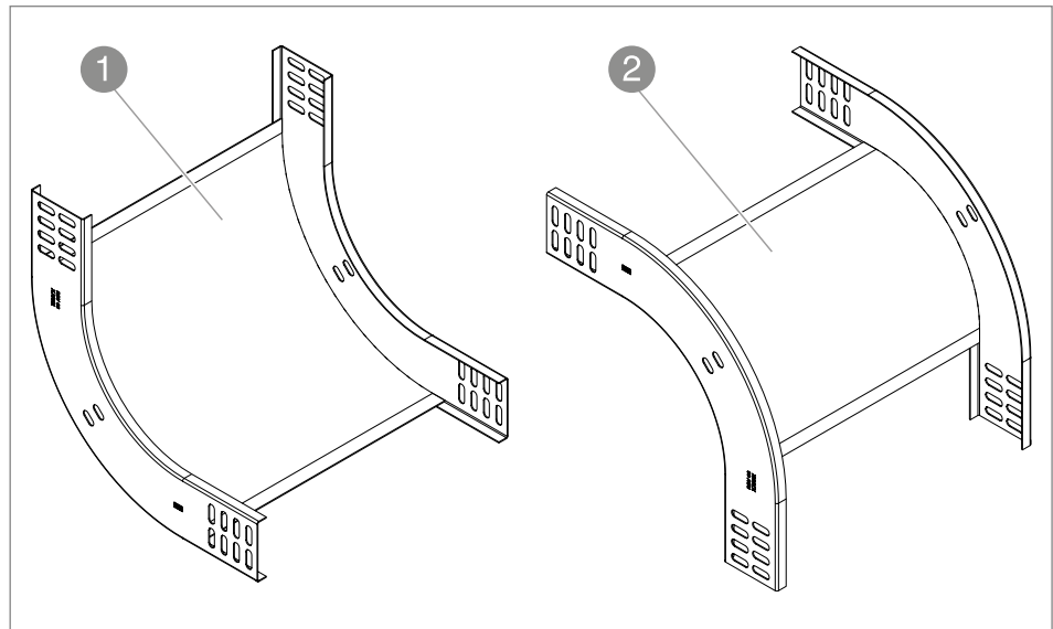
8 pav. kylanti/ besileidžianti vertikaliaji alkūnė
