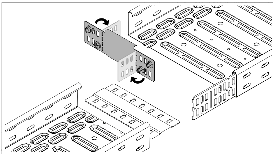
73 pav. Pereinamojo kampinio elemento užlenkimas
