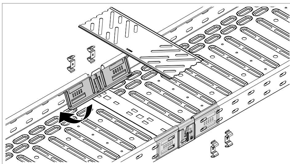
22 pav. Išilginio sujungimo elemento KTSM įstatymas
