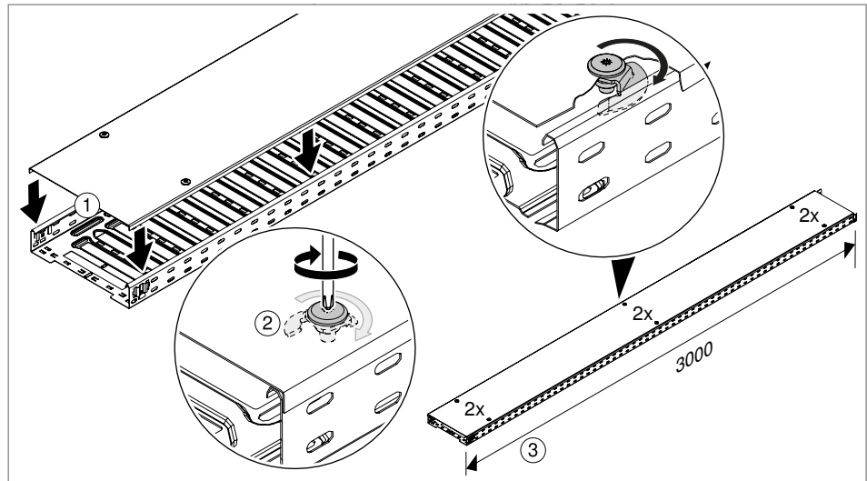
89 pav. Dangčio montavimas spiraline sukamąja sklende
