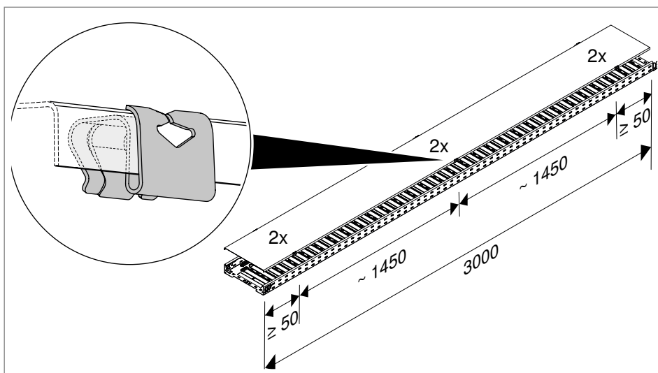
84 pav. Reikiamo dangčio spaustuvių skaičiaus paskirstymas
