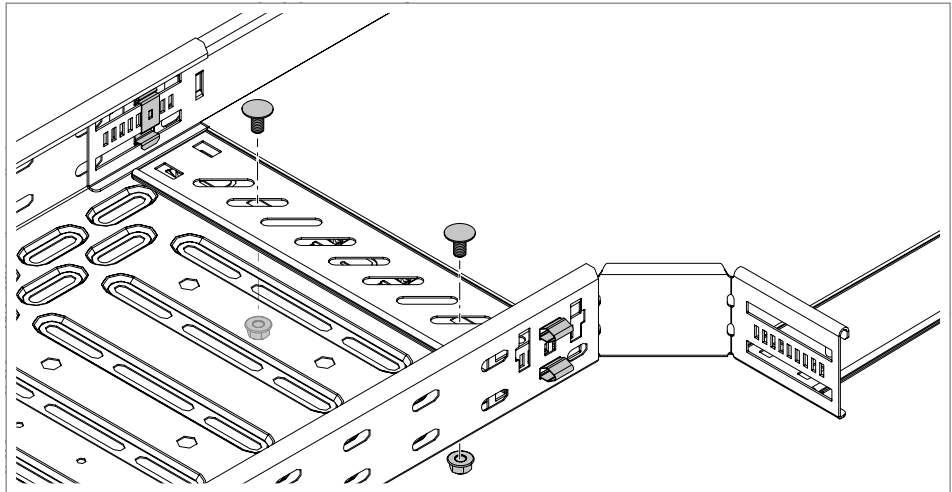
47 pav. Sandūros juostelės prisukimas
