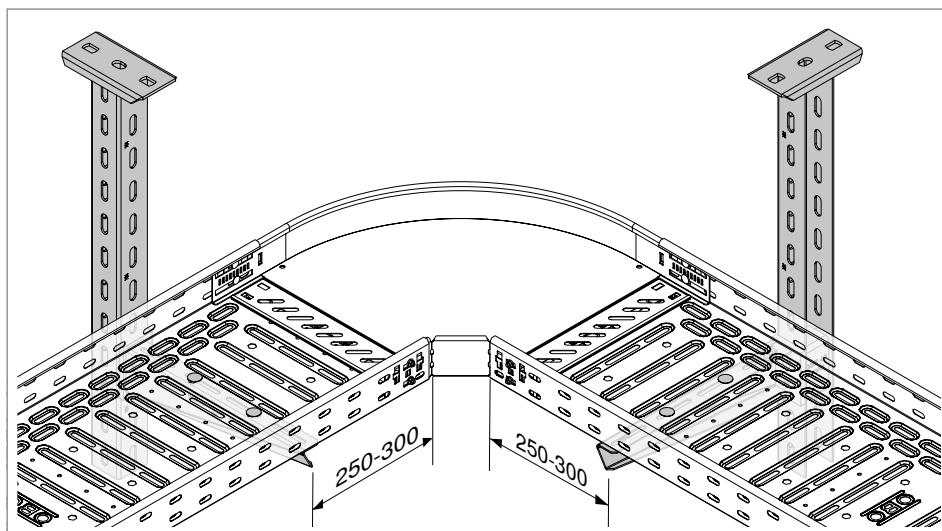
43 pav. 90° alkūnės, 300 mm pločio fasoninės dalies atrėmimo pavyzdys
