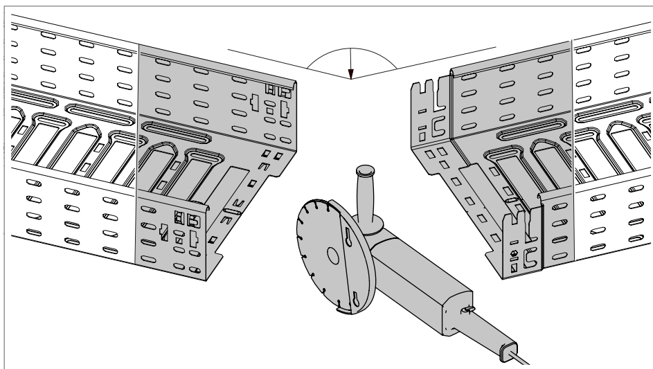
30 pav. Kabelių lovio nupjovimas kampu
