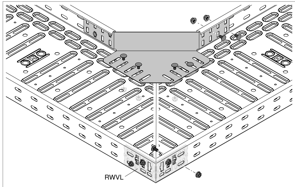
37 pav. Kampo sujungimo elemento REV montavimas
