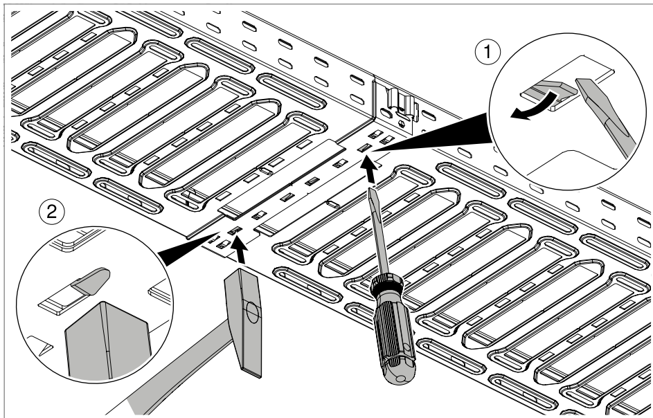
20 pav. Lovių jungties užfiksavimas
