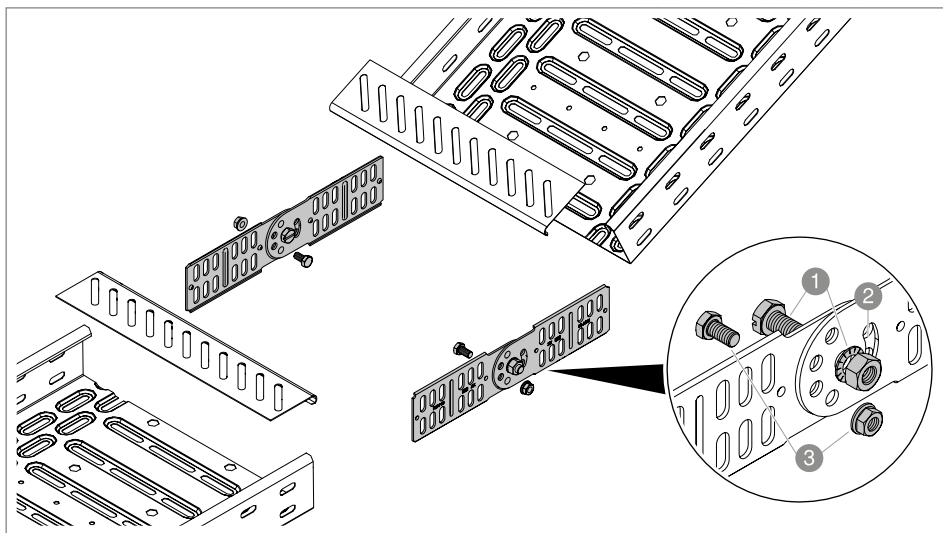
38 pav. Lankstinė jungtis RGV ir pagrindo galinės plokštės
