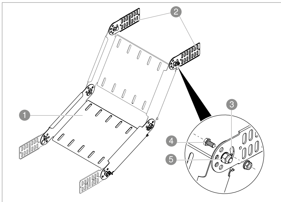
9 pav. Lankstinė alkūnė iš lankstinių alkūnių elementų
