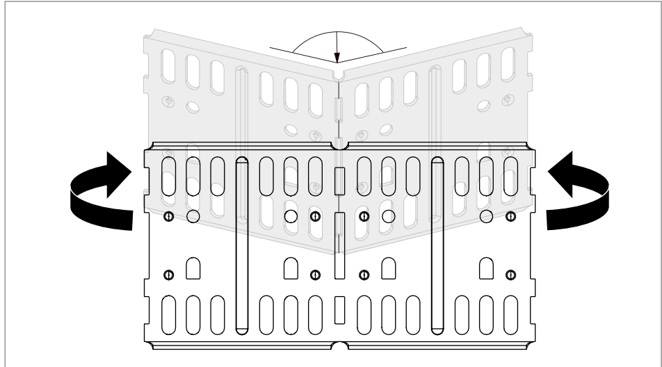
31 pav. Išilginio ir kampinio sujungimo elemento RLVL užlenkimas
