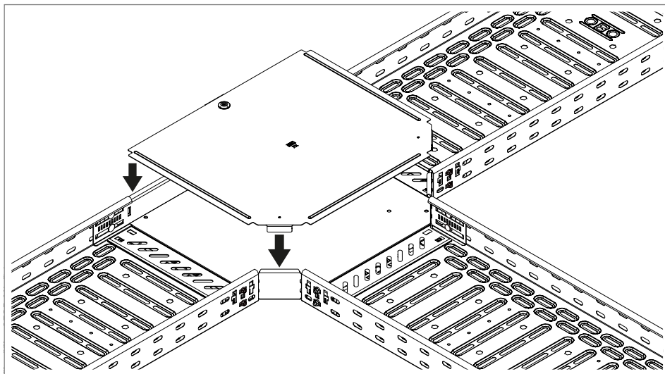
90 pav. Fasoninių dalių dangčio uždėjimas
