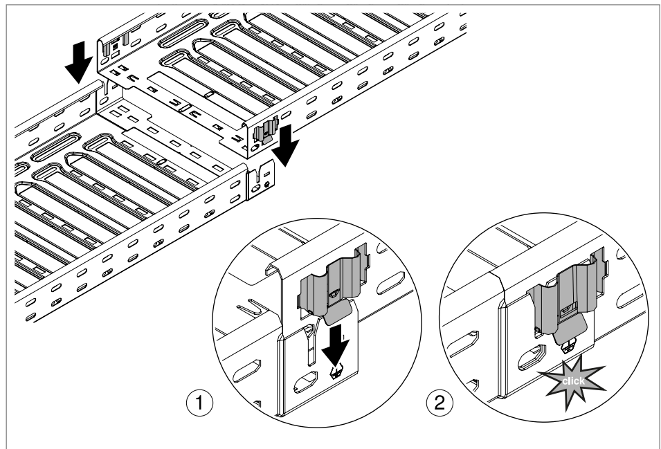
19 pav. Fiksuojamoji jungtis „Magic“ su spyruokliniu elementu
