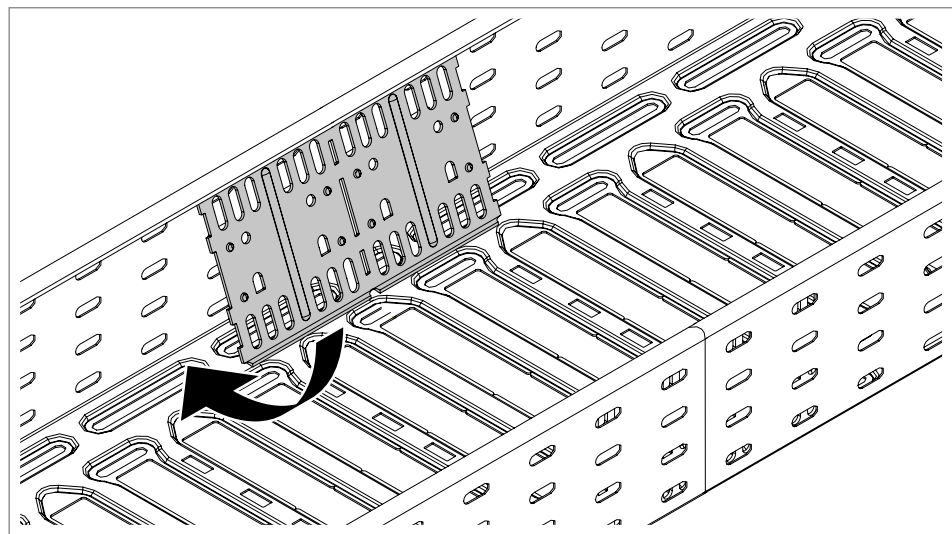
28 pav. Išilginio sujungimo elemento RLVL įstatymas
