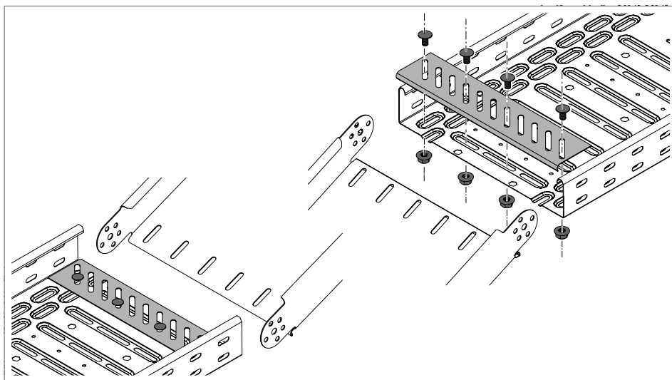
70 pav. Pagrindo galinės plokštės montavimas
