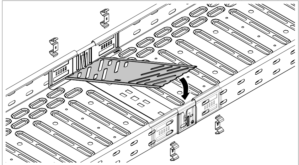
23 pav. Išilginio sujungimo elemento KTSM sandūros juostelės įstatymas
