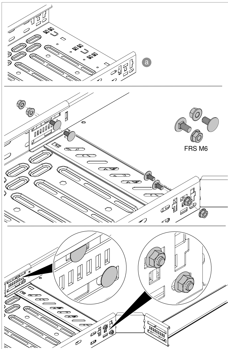
48 pav. Fasoninės dalies pritvirtinimas varžtais (Kabelių lovio galas (a))
