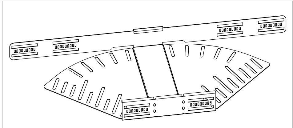
4 pav. Reguliuojamo kampo alkūnės
