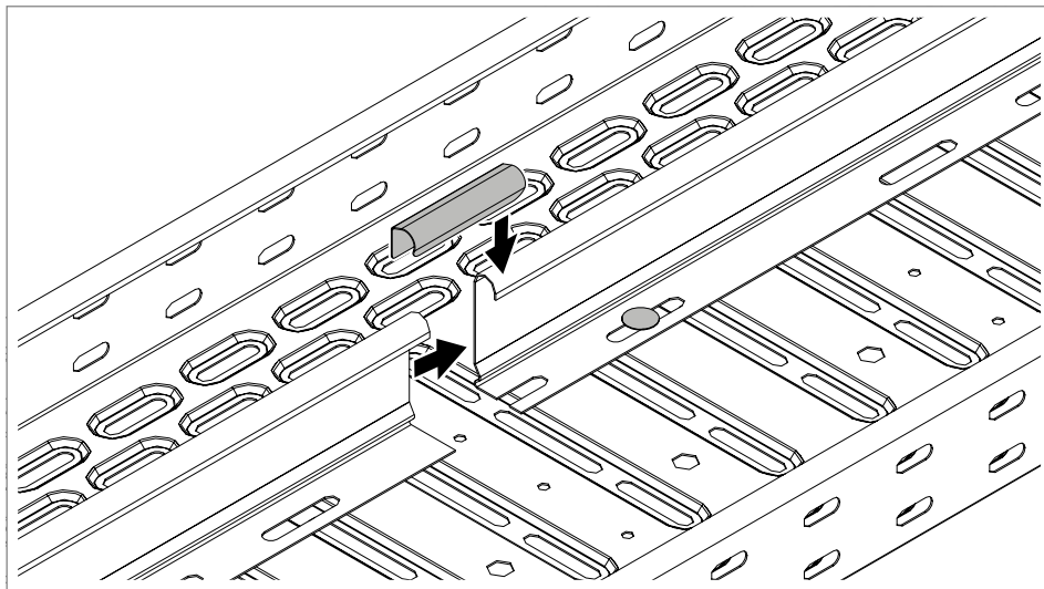
81 pav. Pertvarų sujungimas
