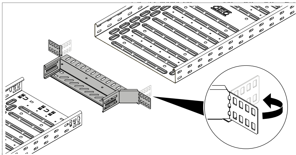
58 pav. Sujungimo plokštelės užlenkimas
