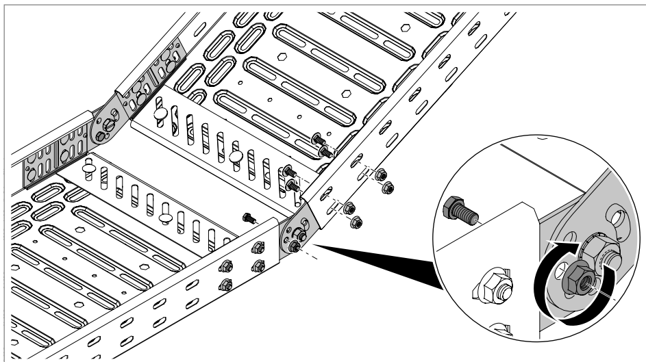
42 pav. Apsauginio varžto priveržimas
