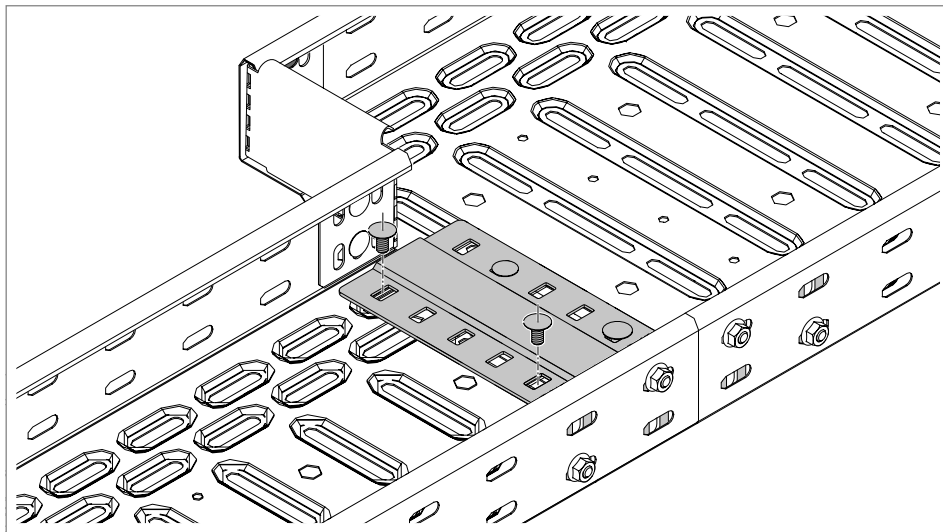
75 pav. Sandūros juostelės prisukimas
