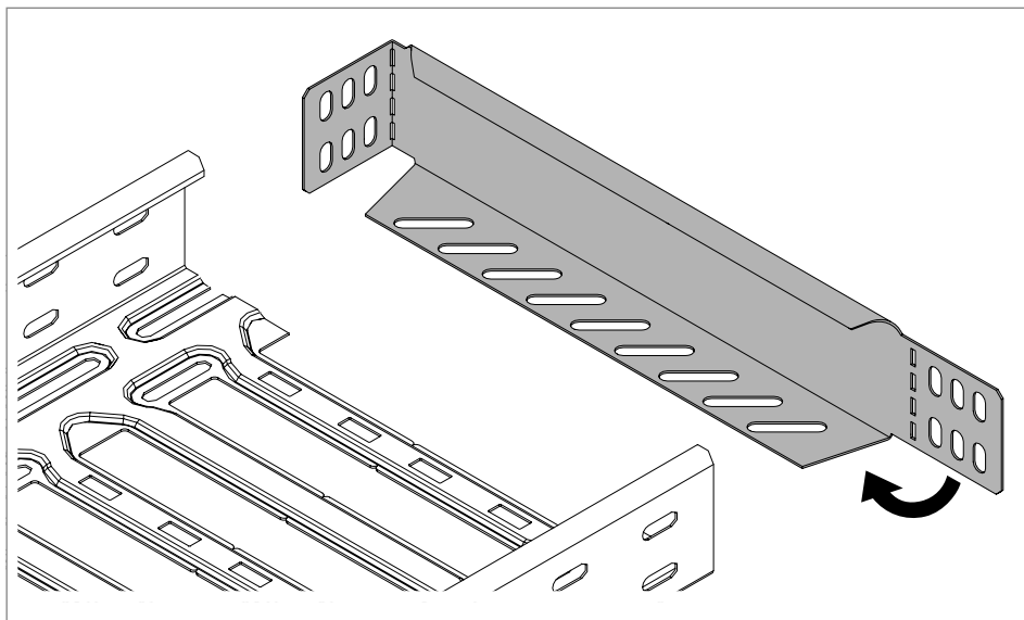
76 pav. Plokštelės užlenkimas
