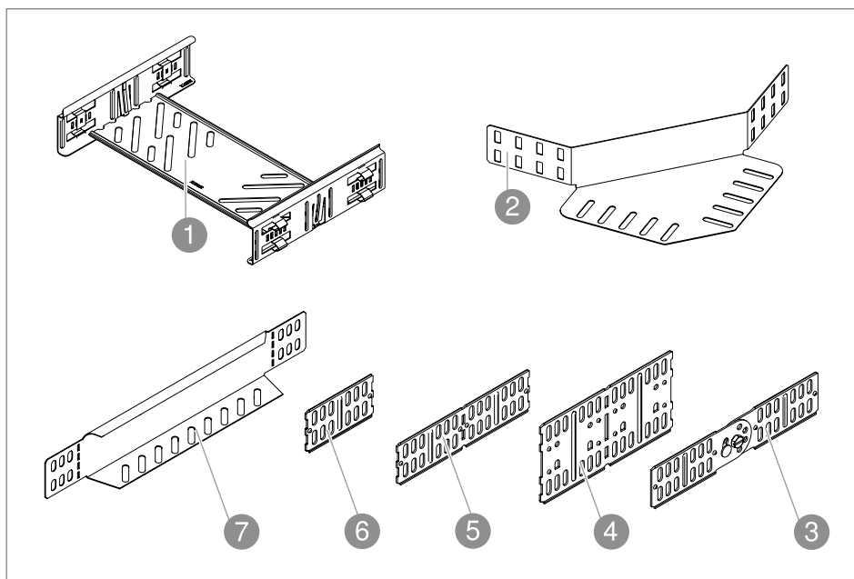
2 pav. Sujungimo elementų apžvalga
