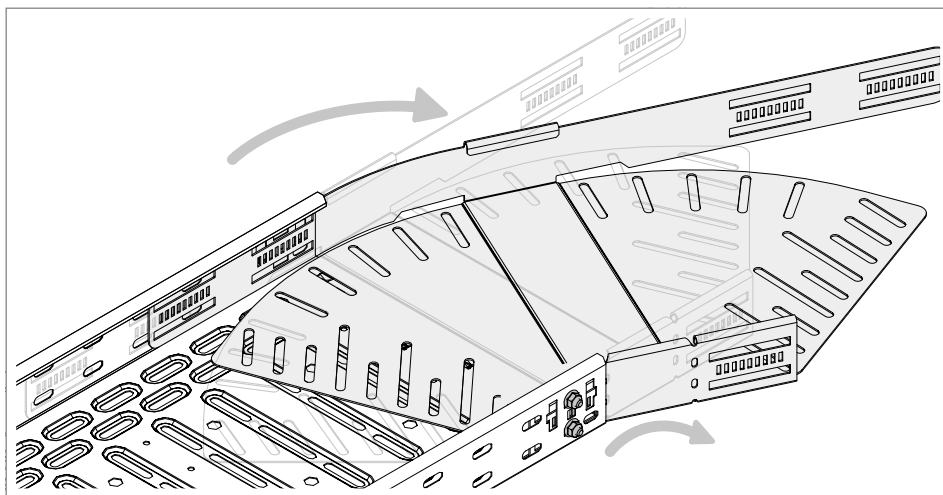
62 pav. Reguliuojamo kampo alkūnės užlenkimas
