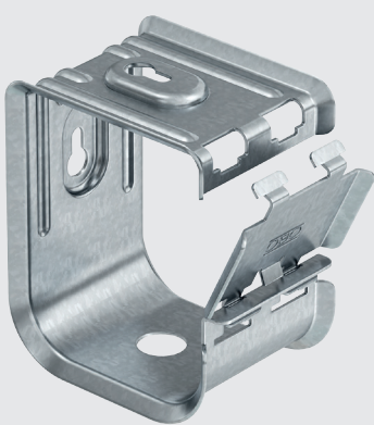
Kabelių laikiklis GRIP M 70 (tipas 2031 M 70)
