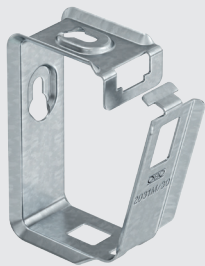
Kabelių laikiklis GRIP M 30 (tipas 2031 M 30)
