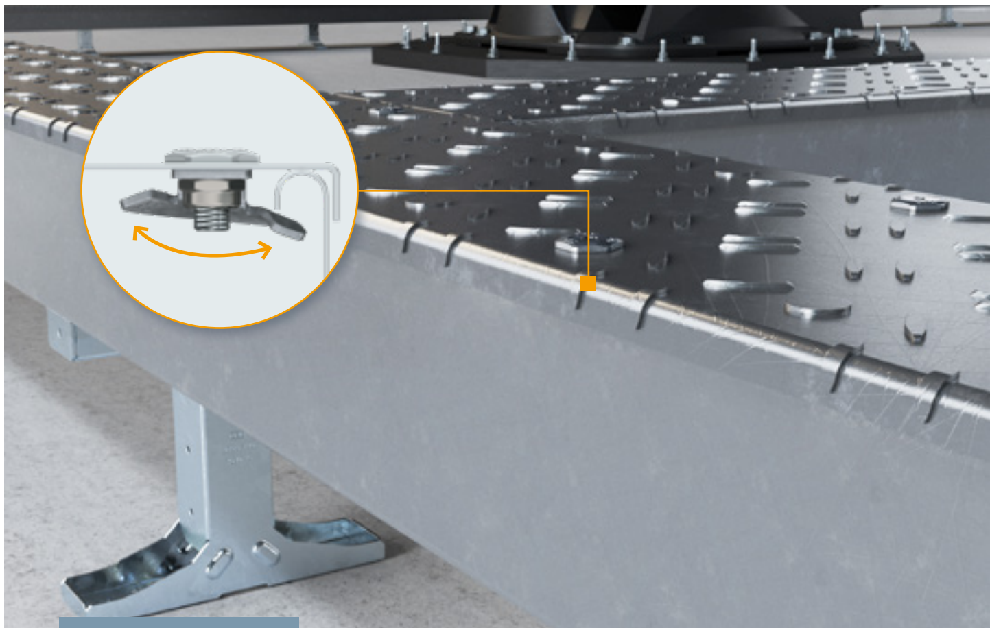
Dangtis su pasukamu užraktu
