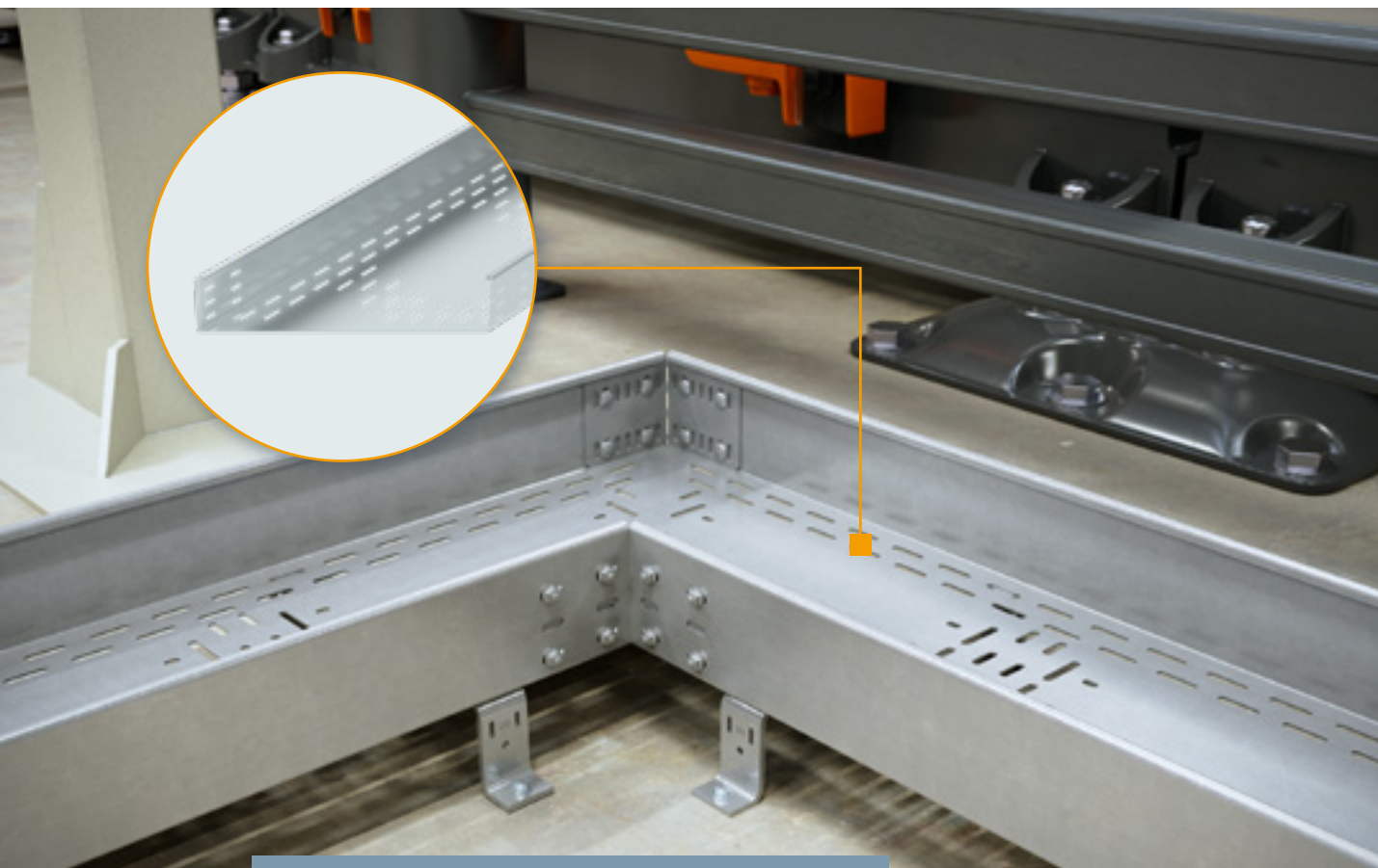
Surenkamieji kanalų ilgiai (1000 mm) su 45 laipsnių kampu
